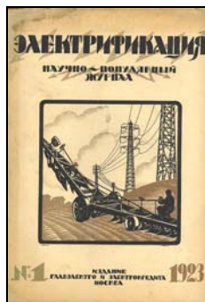
143 Elektrifikazija
